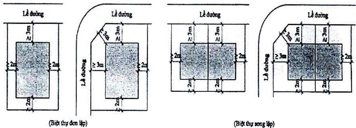
Hình 2.5-Khoảng lùi nhà biệt thự
