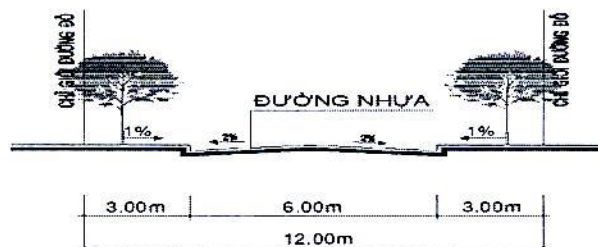
MẶT CẮT NGANG LỘ GIỚI 12M TL:1/100 ( MẶT CẮT 3 - 3 )
