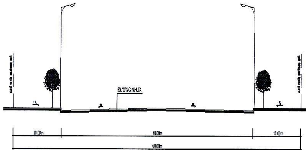
MẶT CẮT NGANG LỘ GIỚI 60M TL:1/100
