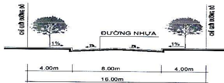
MẶT CẮT NGANG LỘ GIỚI 16M TL:1/100 ( MẶT CẮT 7 - 7 )
