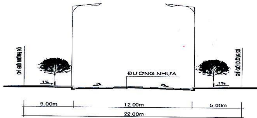
MẶT CẮT NGANG LỘ GIỚI 22M TL:1/100 ( MẶT CẮT 2 - 2 )
