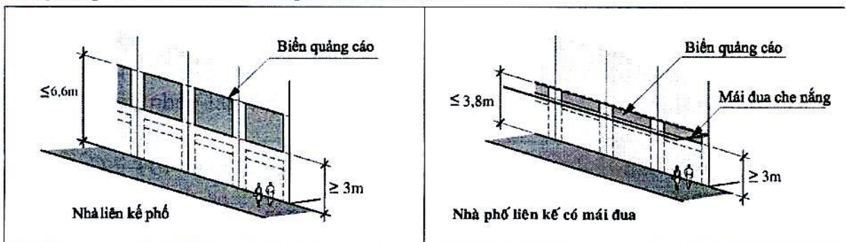
Hình 2.6-Quy định quảng cáo đối với nhà liên kế phố
