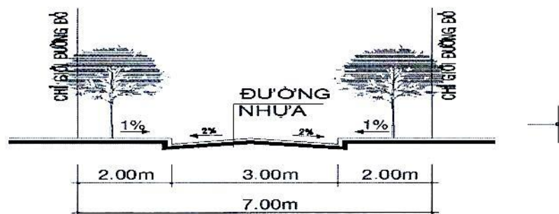
MẶT CẮT NGANG LỘ GIỚI 7M ( MẶT CẮT 8 - 8 )
