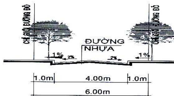
MẶT CẮT NGANG LỘ GIỚI 6M ( MẶT CẮT 11 - 11 )
