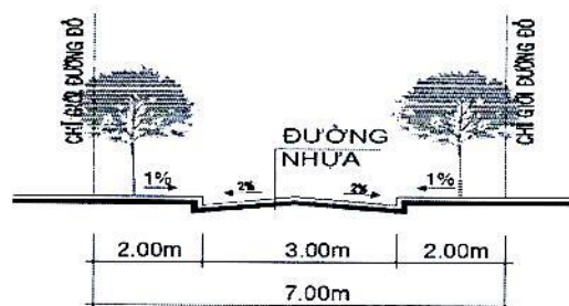
MẶT CẮT NGANG LỘ GIỚI 7M TL:1/100 ( MẶT CẮT 9 - 9 )
